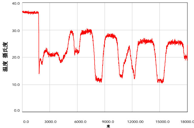
DTS Manager 软件典型的温度跟踪
