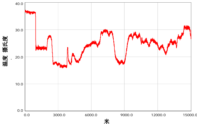
DTS Manager 软件典型的温度跟踪
